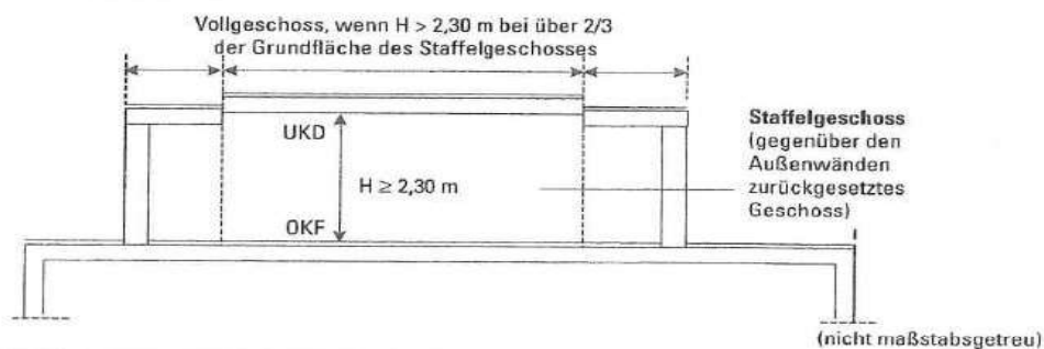
3. Abb.: Staffelgeschoss mit Flachdach
