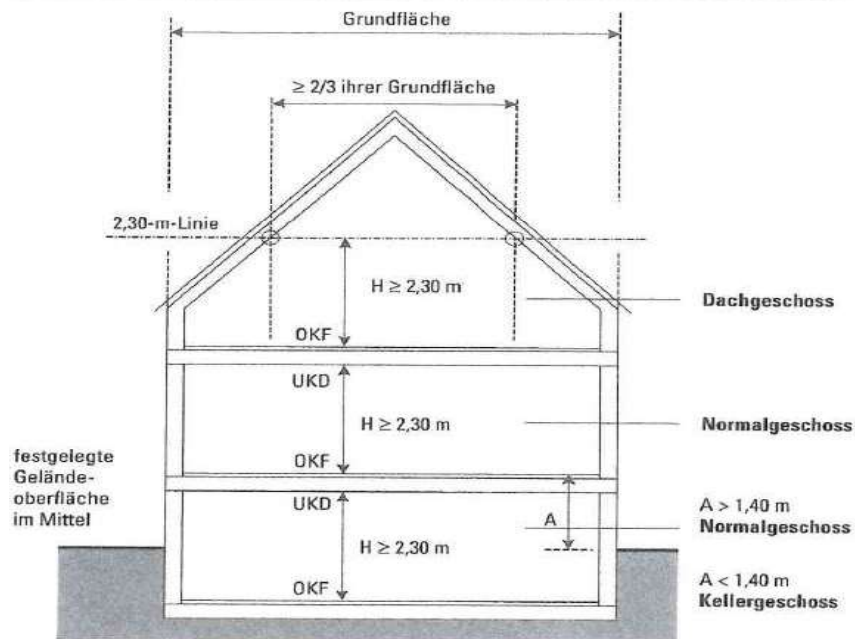
2. Abb: schematische Darstellung von Geschosstypen mit Satteldach
