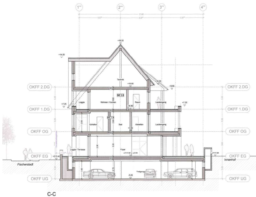
2. Abb: schematische Darstellung von Geschosstypen mit Satteldach
